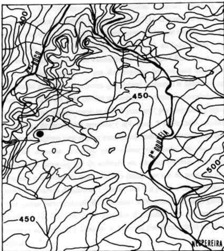
Fig.2- Implantação do Penedo dos Mouros (escala 1 :25 000)
