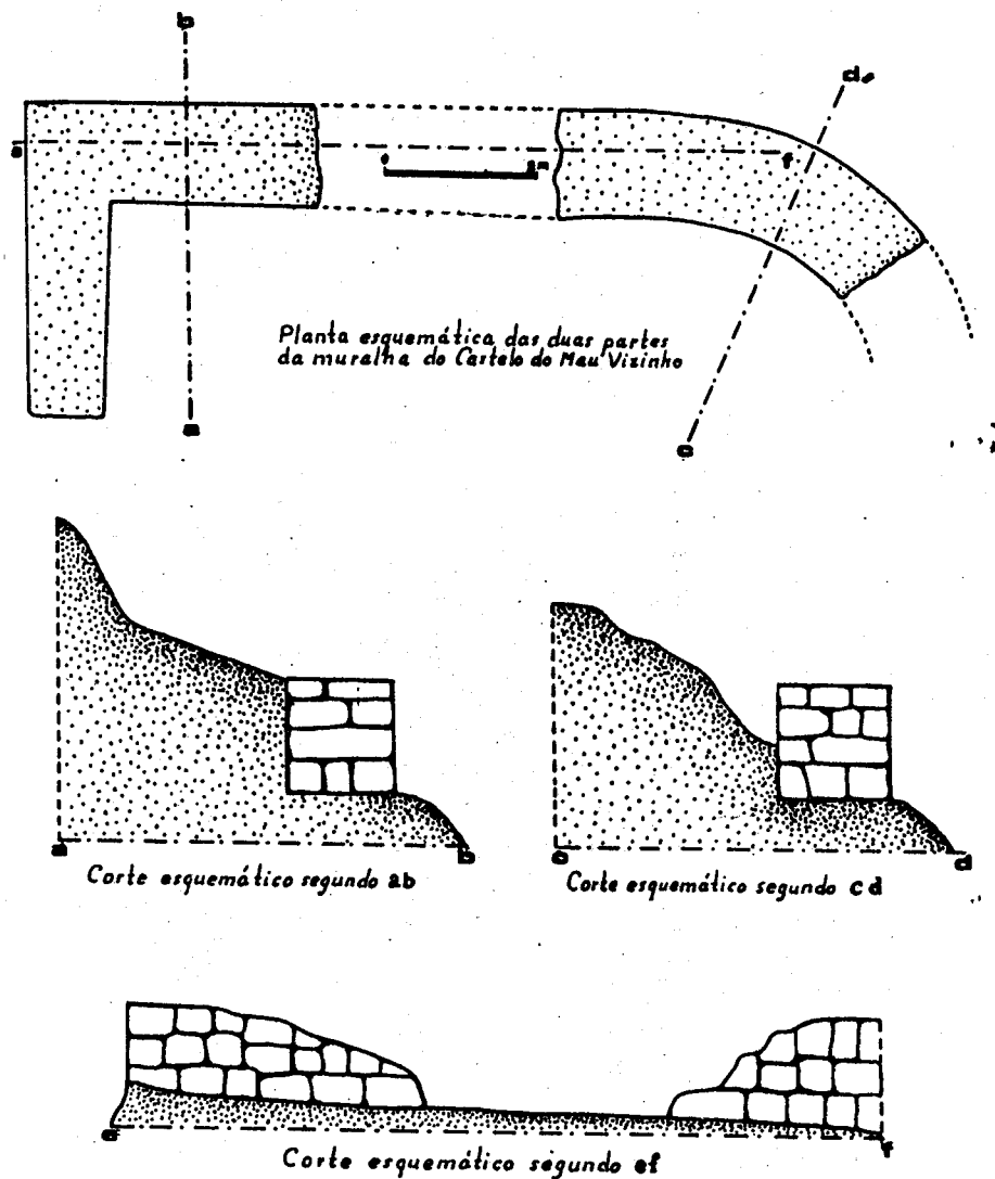
Fig. 9 — Esquema dos dois troços da muralha envolvente do recinto central e respectivos cortes segundo ab e cd .
