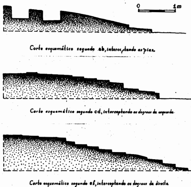
Fig. 4 — Cortes esquemáticos (direcção E-W) das cavidades e das duas séries de degraus.
