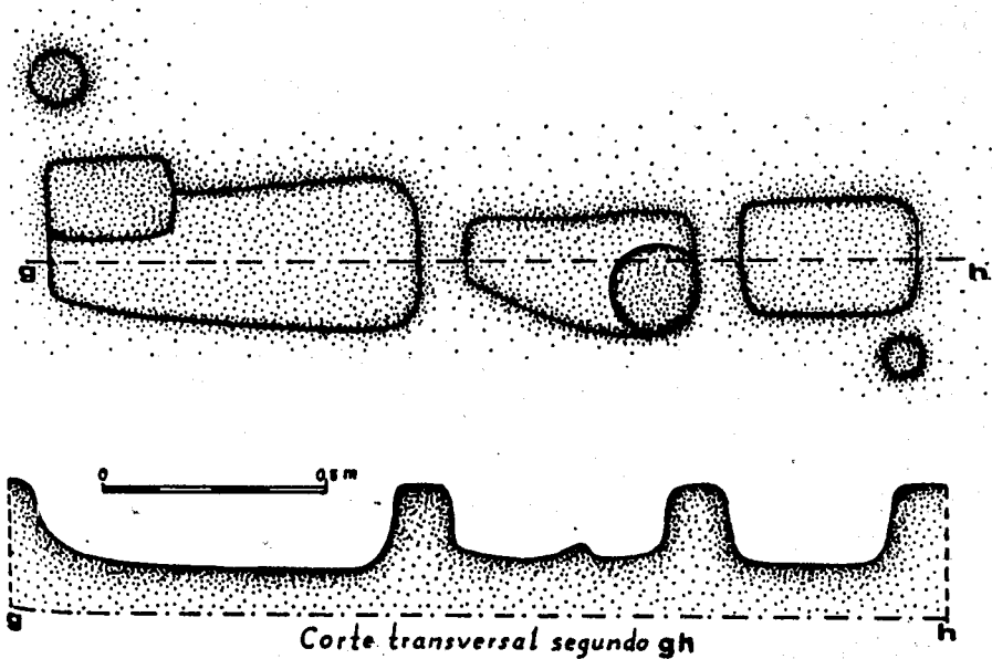
Fig. 6 — Posição relativa de algumas das cavidades de maiores dimensões do recinto central do santuário.
