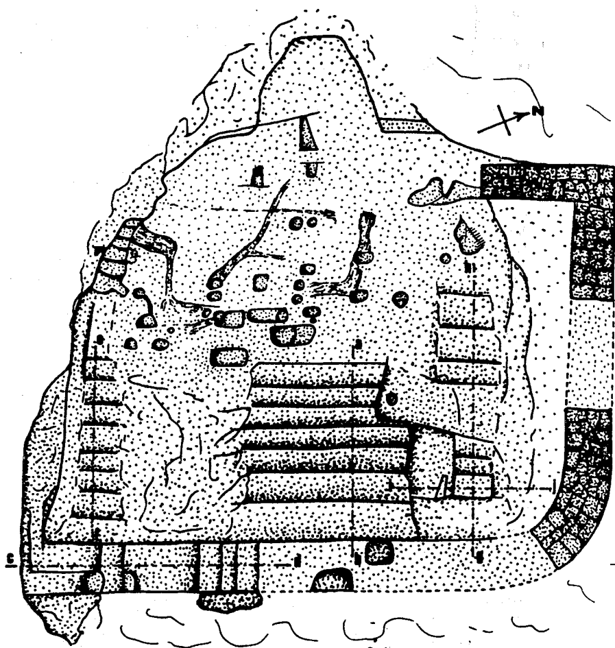
Fig. 5 — Planta esquemática do topo cimeiro do santuário, indicando a posição do muro envolvente, dos degraus e de algumas cavidades e sulcos.
