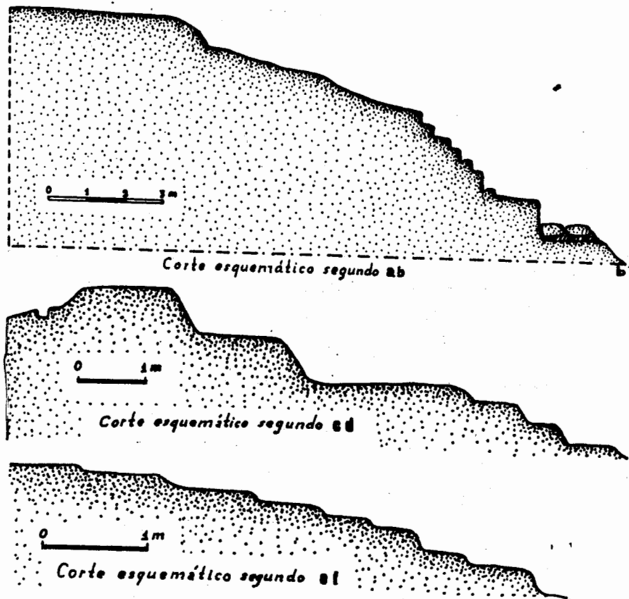
Fig. 7 — Cortes esquemáticos (fig. 5) segundo ab , cd e ef .
