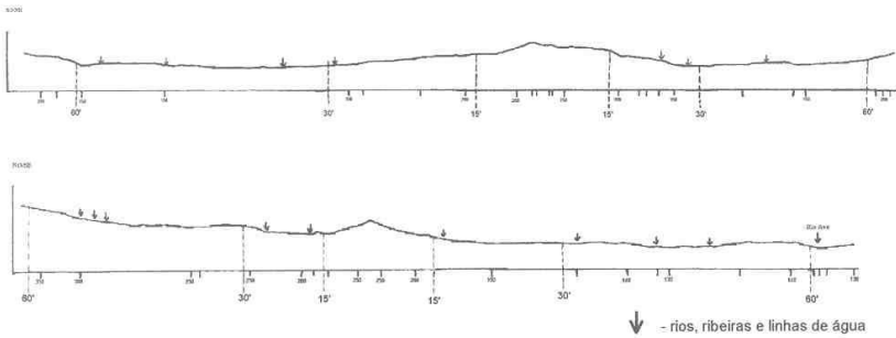
Fig. 2 - Perfis topográficos do castro de Sabroso
